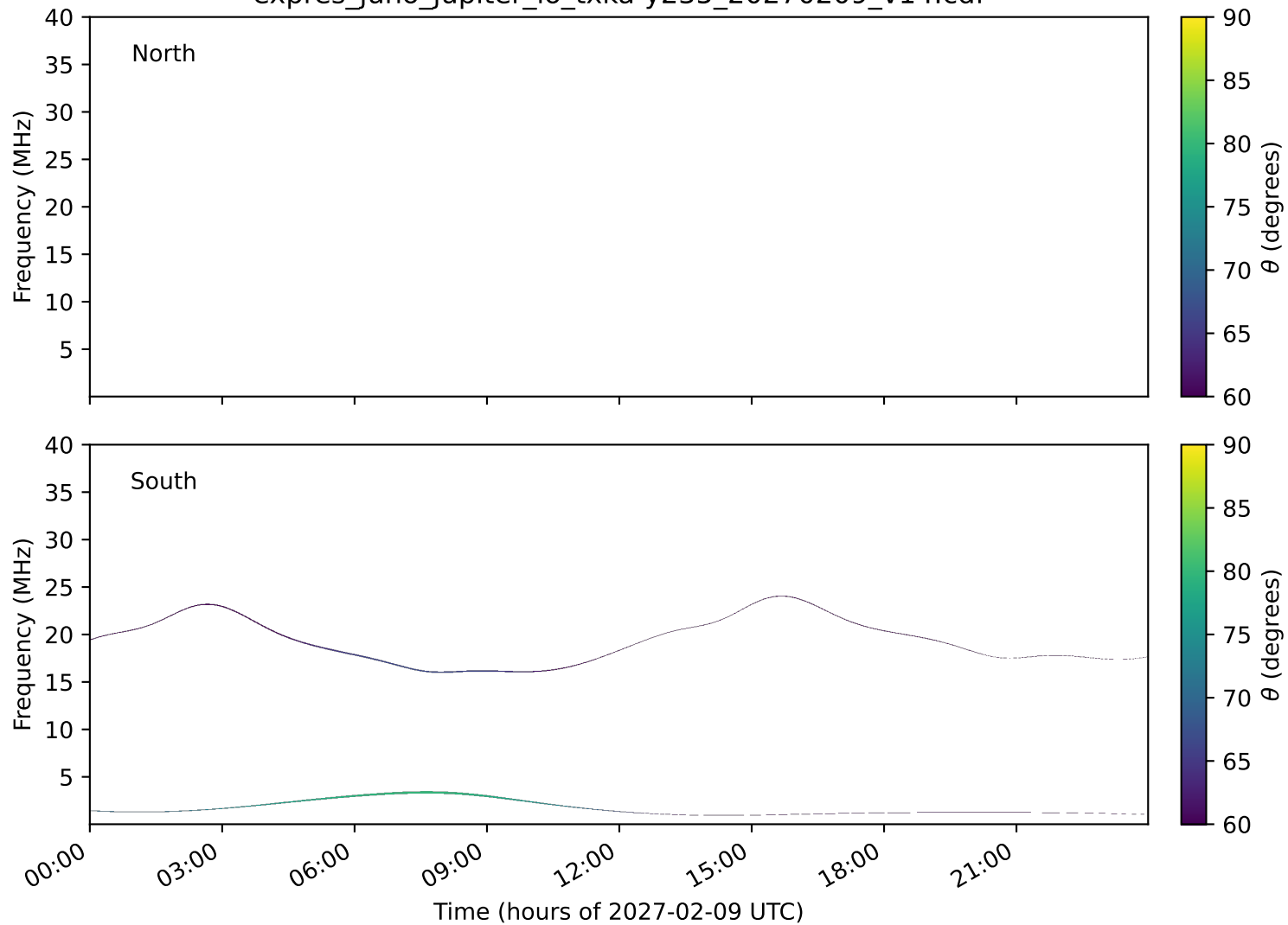
expres_juno_jupiter_io_txka-y235_20270209_v14.cdf
