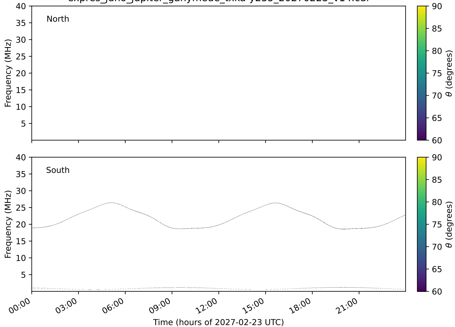
expres_juno_jupiter_ganymede_txka-y235_20270223_v14.cdf
