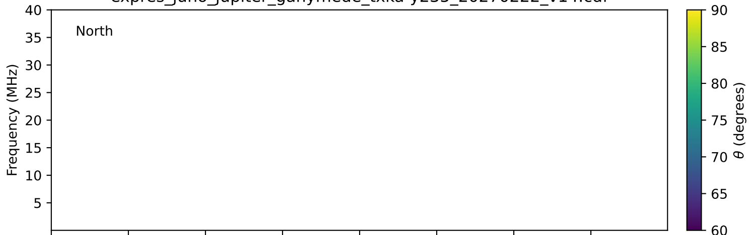
expres_juno_jupiter_ganymede_txka-y235_20270222_v14.cdf
