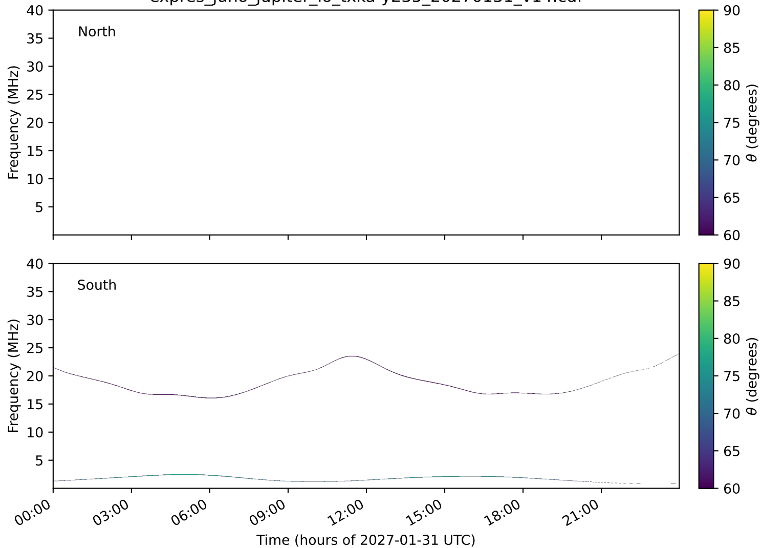
expres_juno_jupiter_io_txka-y235_20270131_v14.cdf
