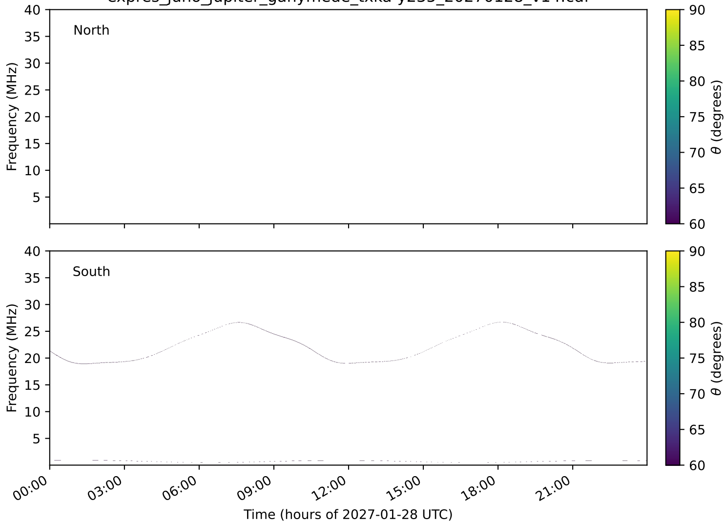
expres_juno_jupiter_ganymede_txka-y235_20270128_v14.cdf
