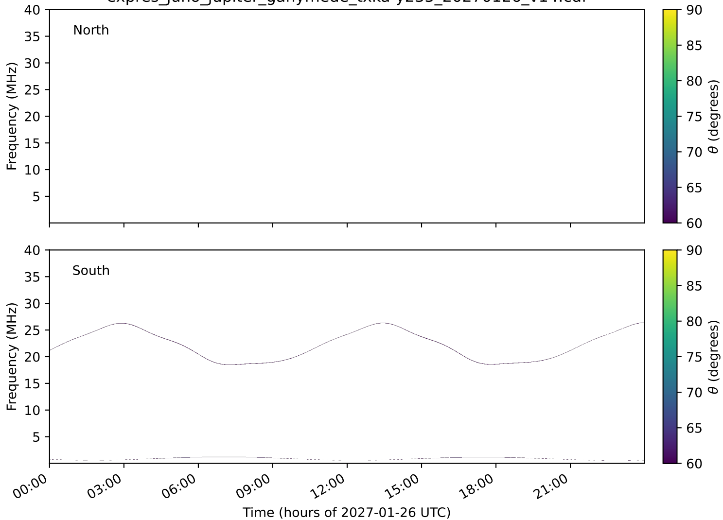
expres_juno_jupiter_ganymede_txka-y235_20270126_v14.cdf
