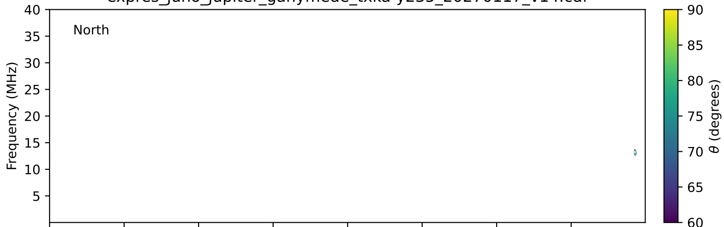
expres_juno_jupiter_ganymede_txka-y235_20270117_v14.cdf
