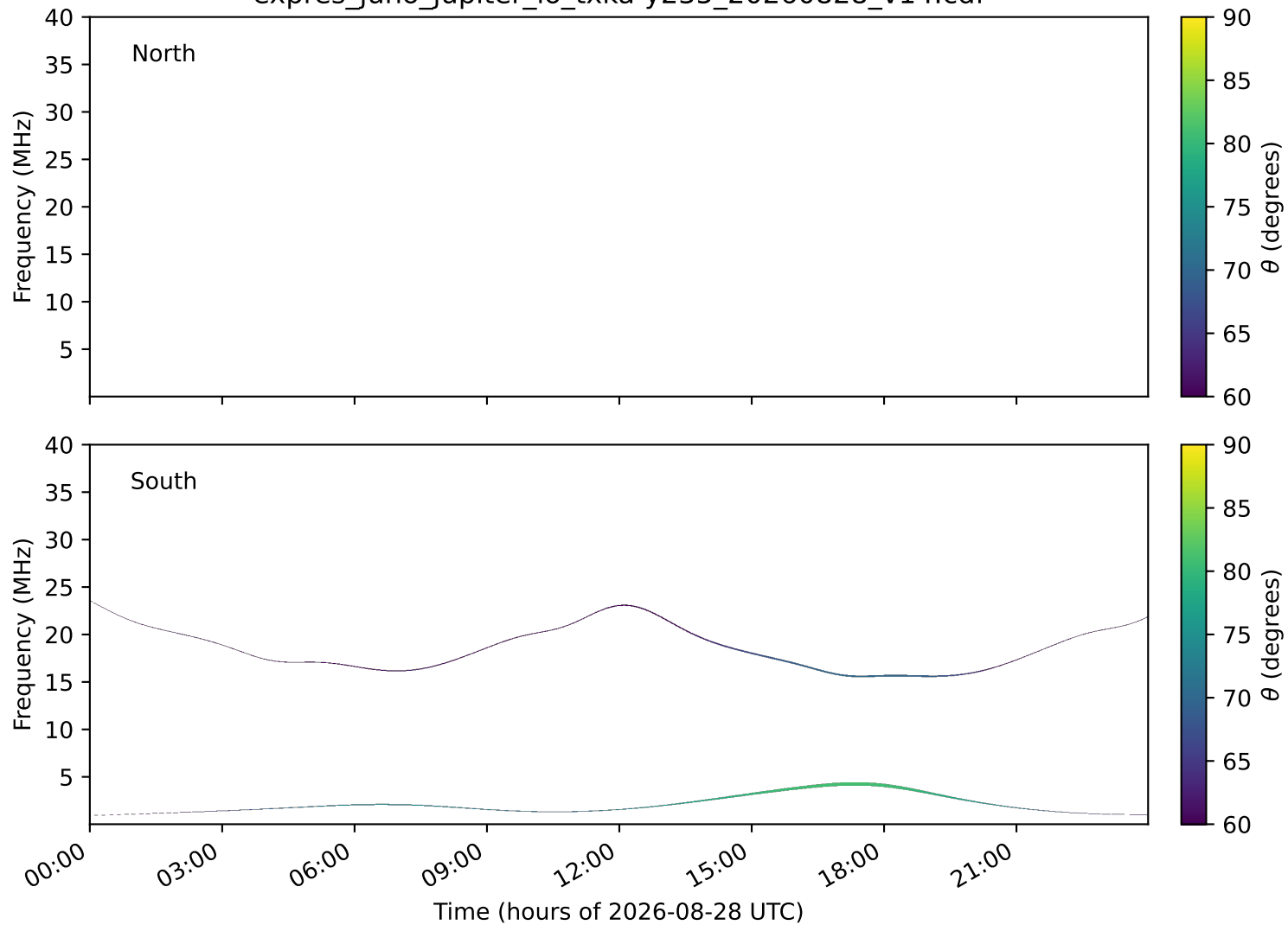
expres_juno_jupiter_io_txka-y235_20260828_v14.cdf
