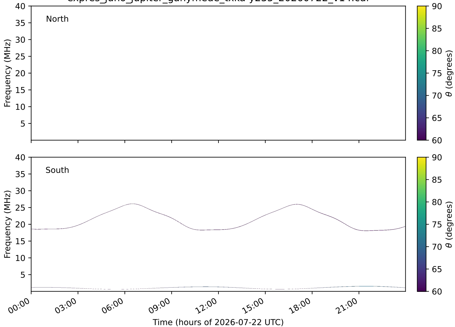
expres_juno_jupiter_ganymede_txka-y235_20260722_v14.cdf
