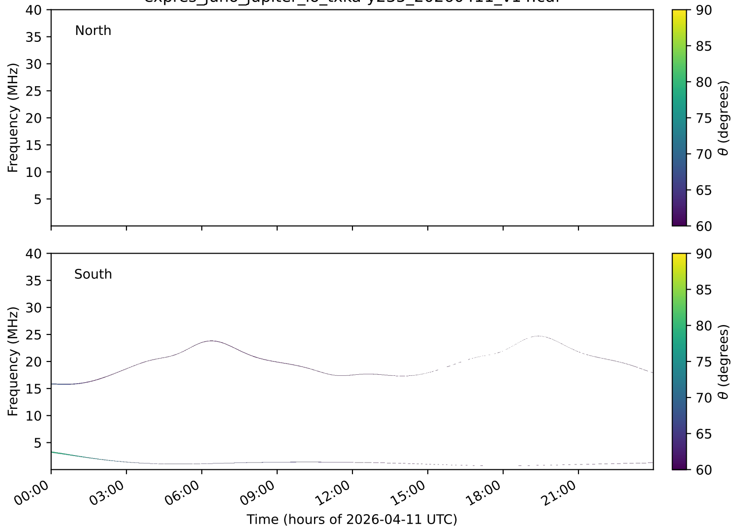
expres_juno_jupiter_io_txka-y235_20260411_v14.cdf
