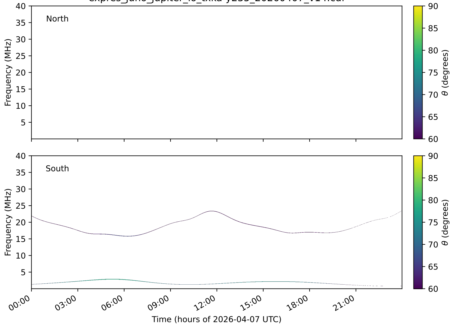
expres_juno_jupiter_io_txka-y235_20260407_v14.cdf
