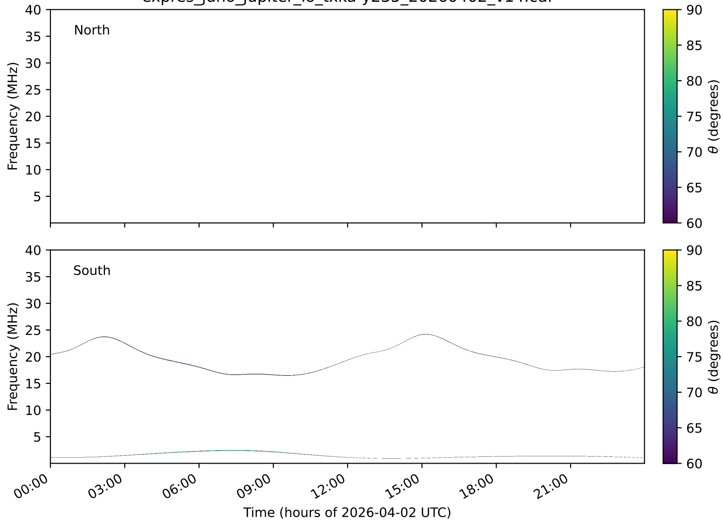
expres_juno_jupiter_io_txka-y235_20260402_v14.cdf
