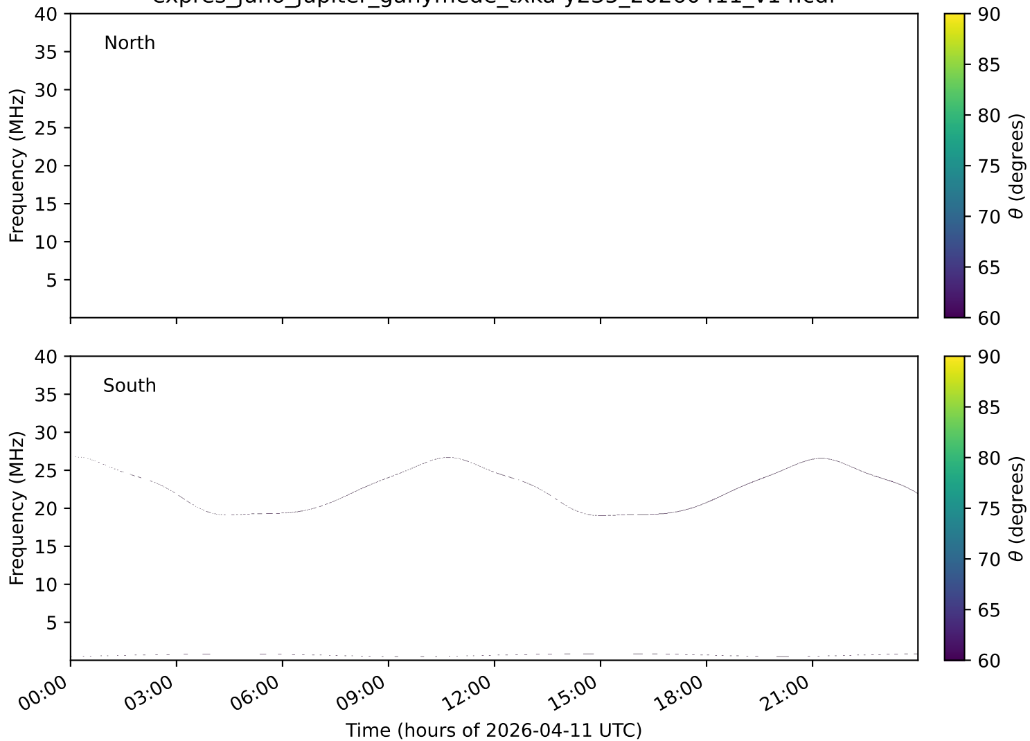
expres_juno_jupiter_ganymede_txka-y235_20260411_v14.cdf
