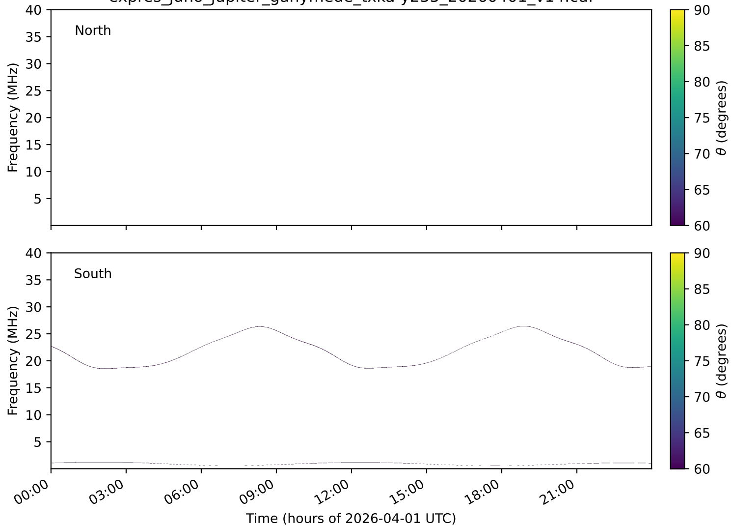
expres_juno_jupiter_ganymede_txka-y235_20260401_v14.cdf
