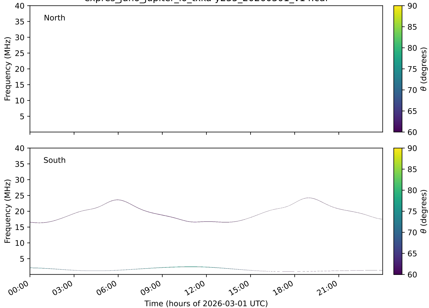
expres_juno_jupiter_io_txka-y235_20260301_v14.cdf
