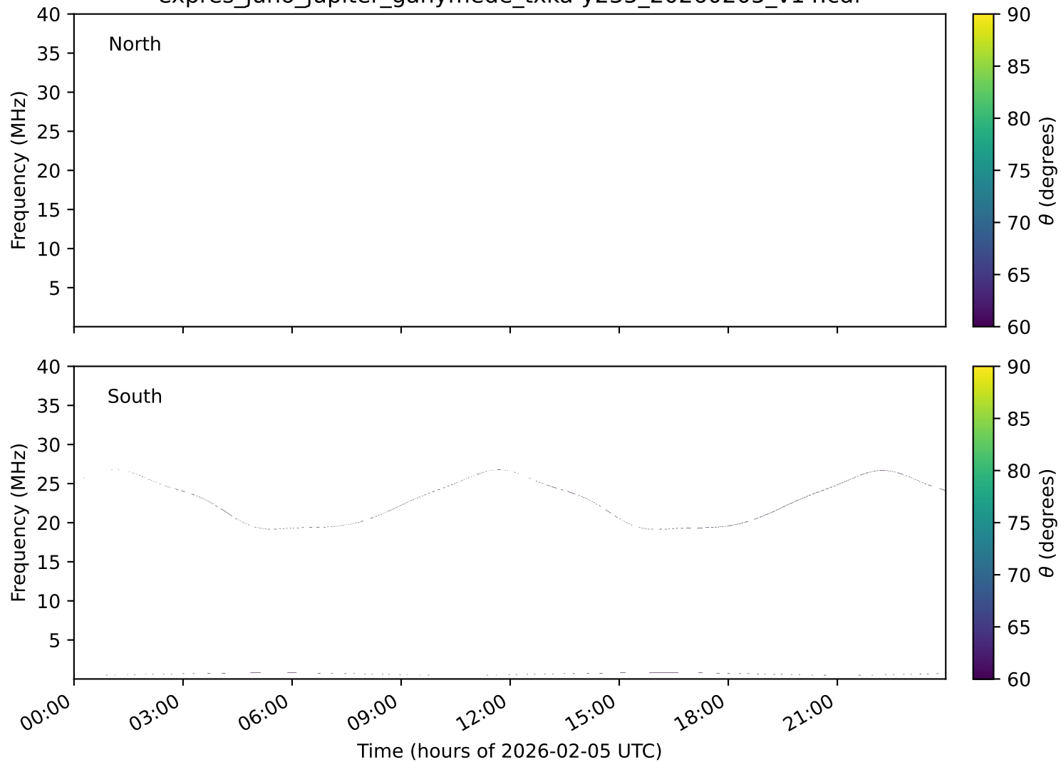
expres_juno_jupiter_ganymede_txka-y235_20260205_v14.cdf
