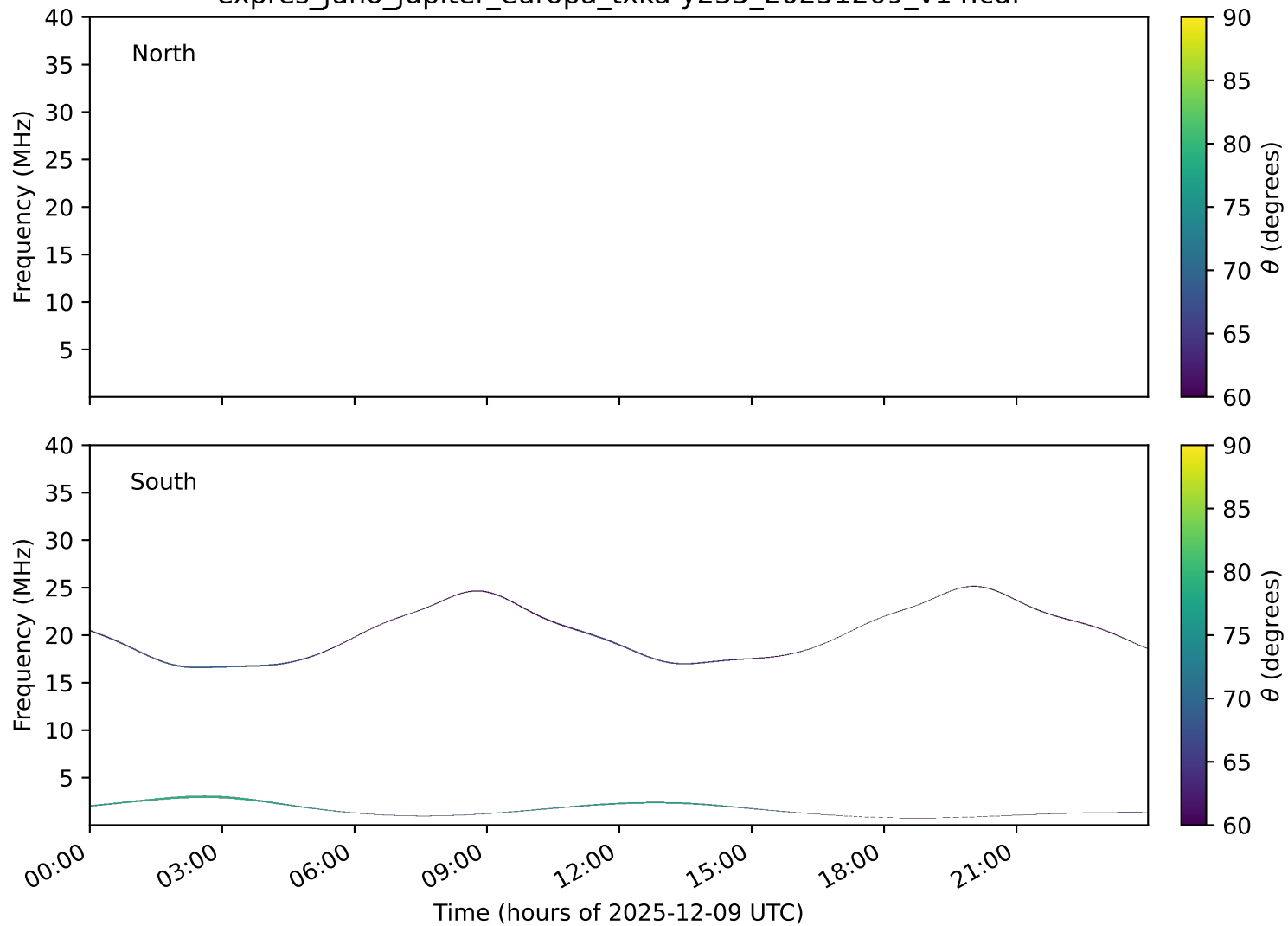
expres_juno_jupiter_europa_txka-y235_20251209_v14.cdf
