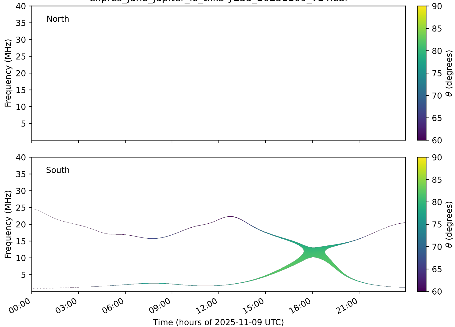
expres_juno_jupiter_io_txka-y235_20251109_v14.cdf
