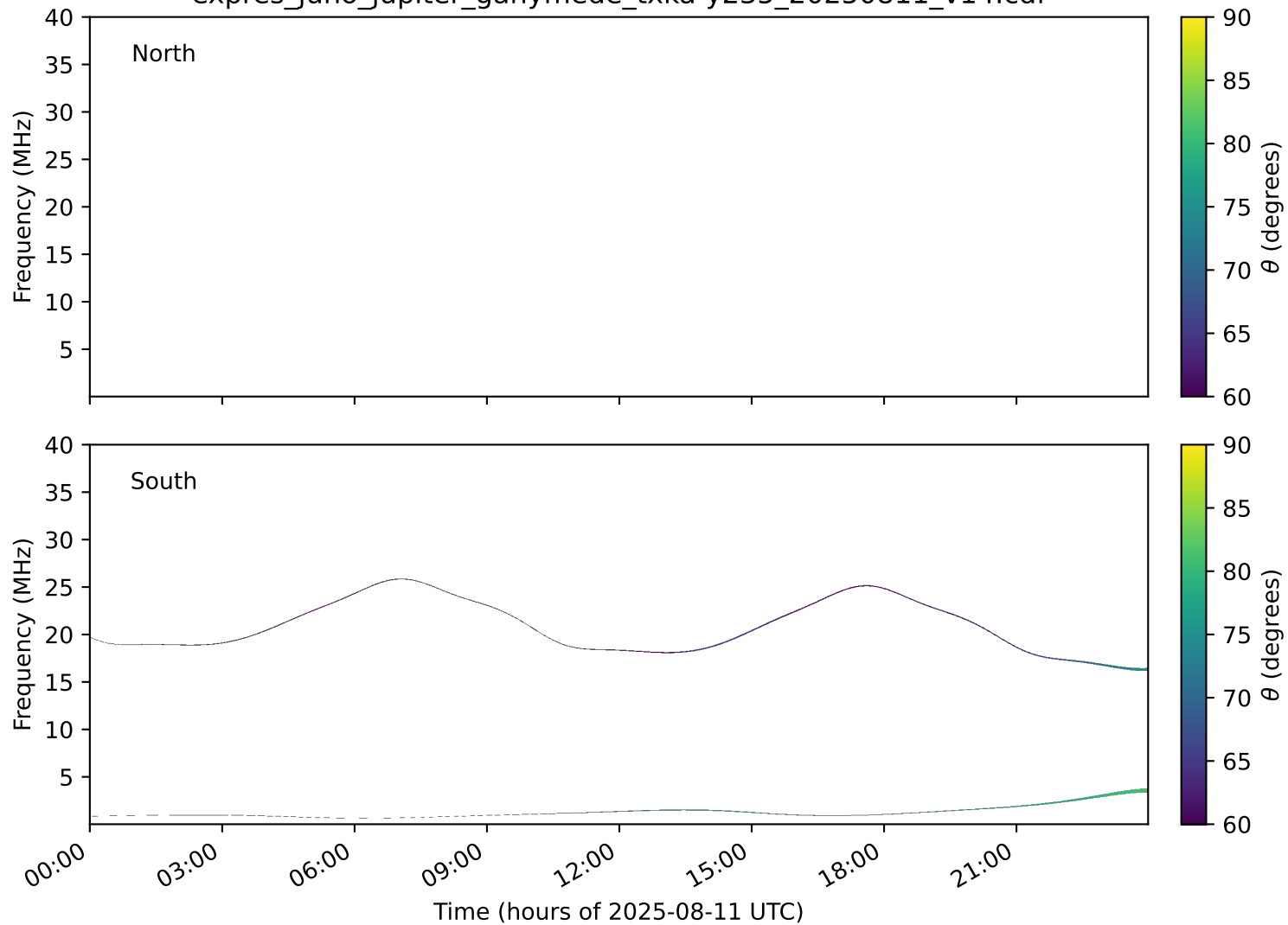
expres_juno_jupiter_ganymede_txka-y235_20250811_v14.cdf
