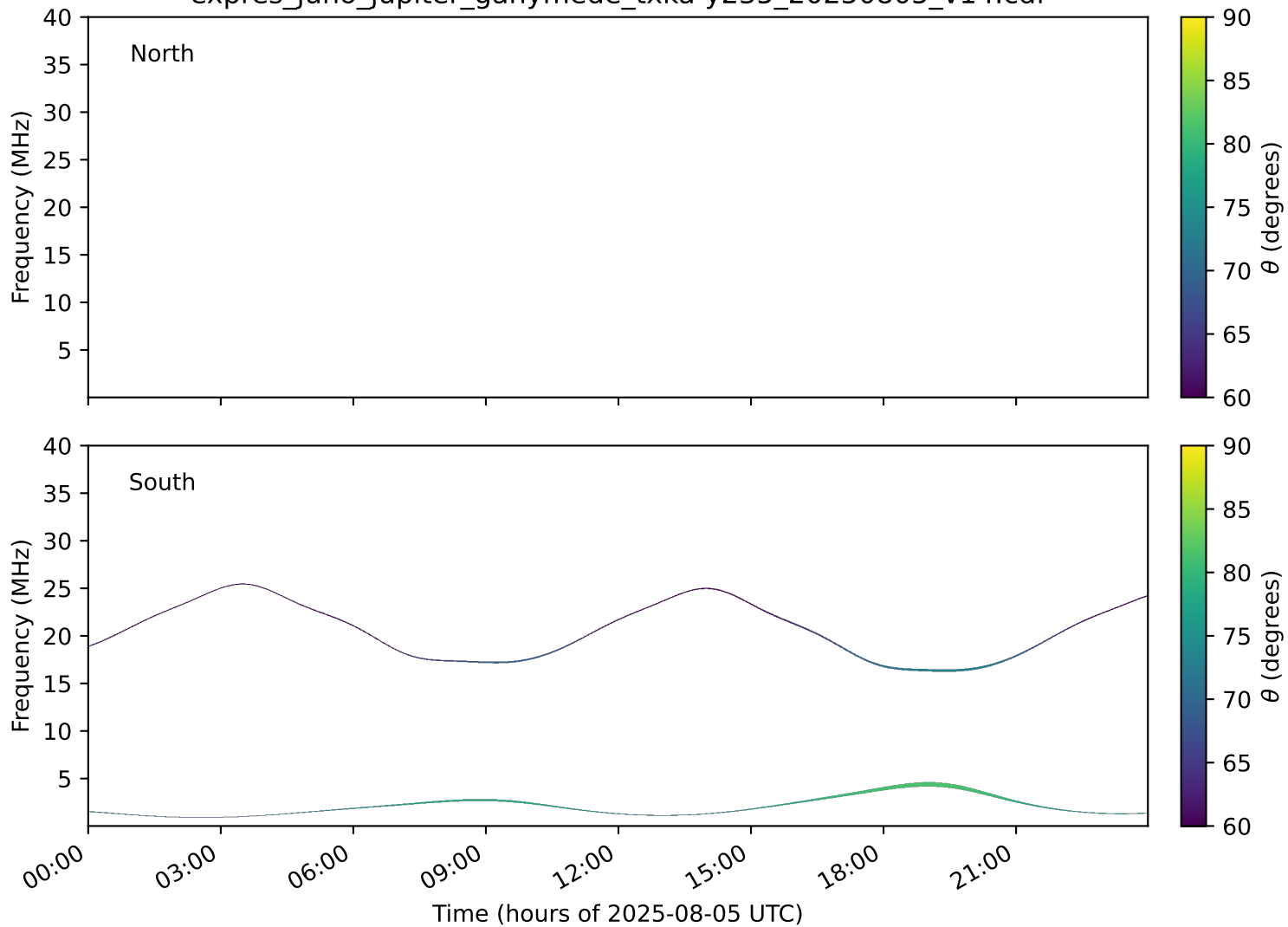
expres_juno_jupiter_ganymede_txka-y235_20250805_v14.cdf
