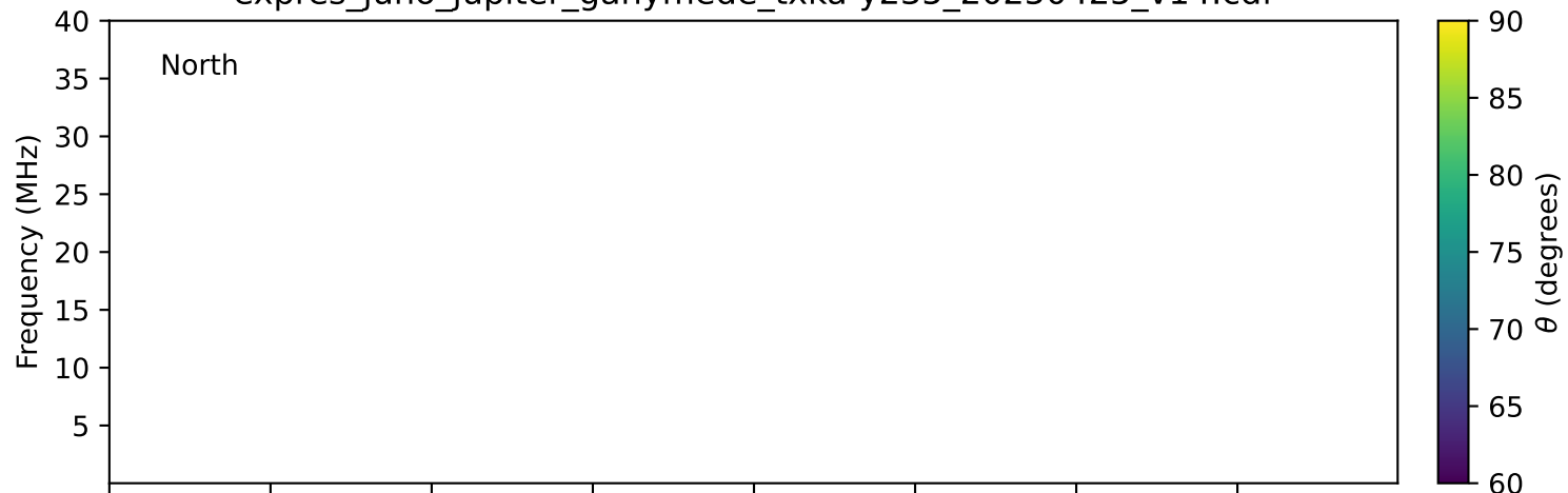
expres_juno_jupiter_ganymede_txka-y235_20250425_v14.cdf
