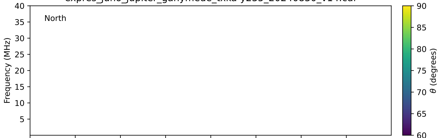
expres_juno_jupiter_ganymede_txka-y235_20240830_v14.cdf
