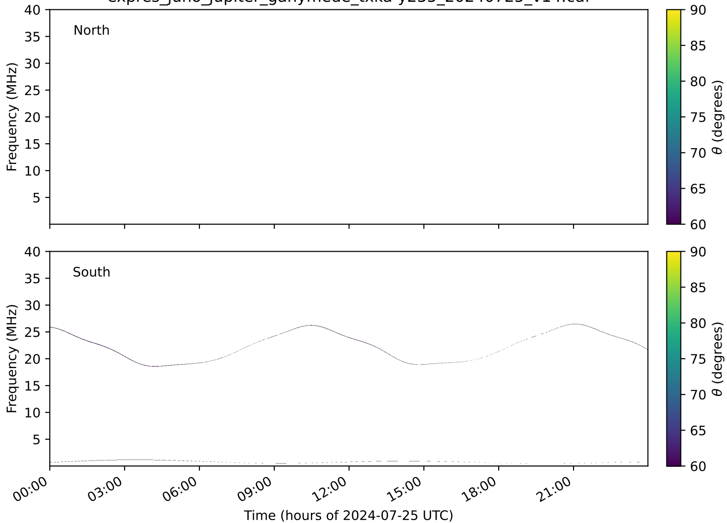
expres_juno_jupiter_ganymede_txka-y235_20240725_v14.cdf
