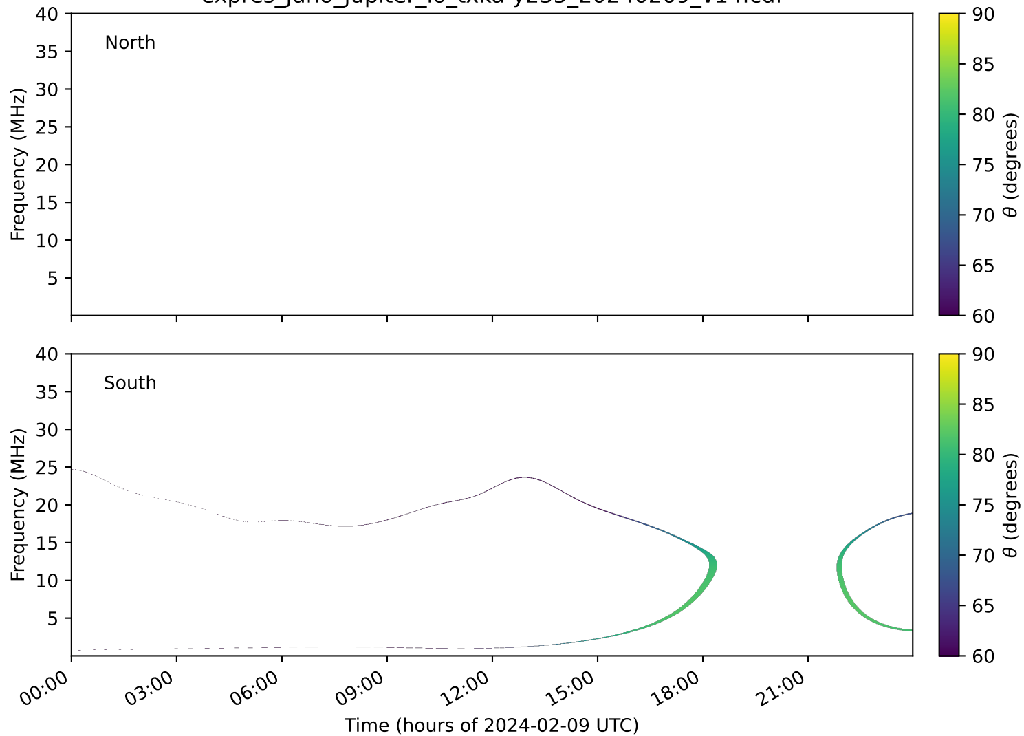
expres_juno_jupiter_io_txka-y235_20240209_v14.cdf
