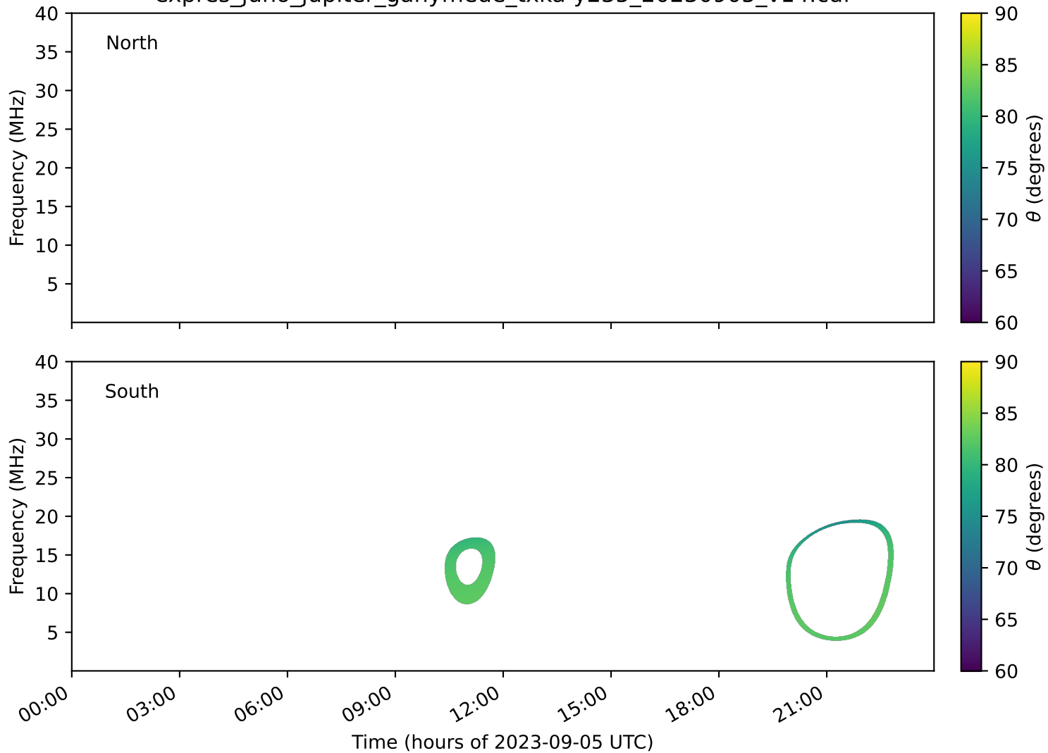
expres_juno_jupiter_ganymede_txka-y235_20230905_v14.cdf
