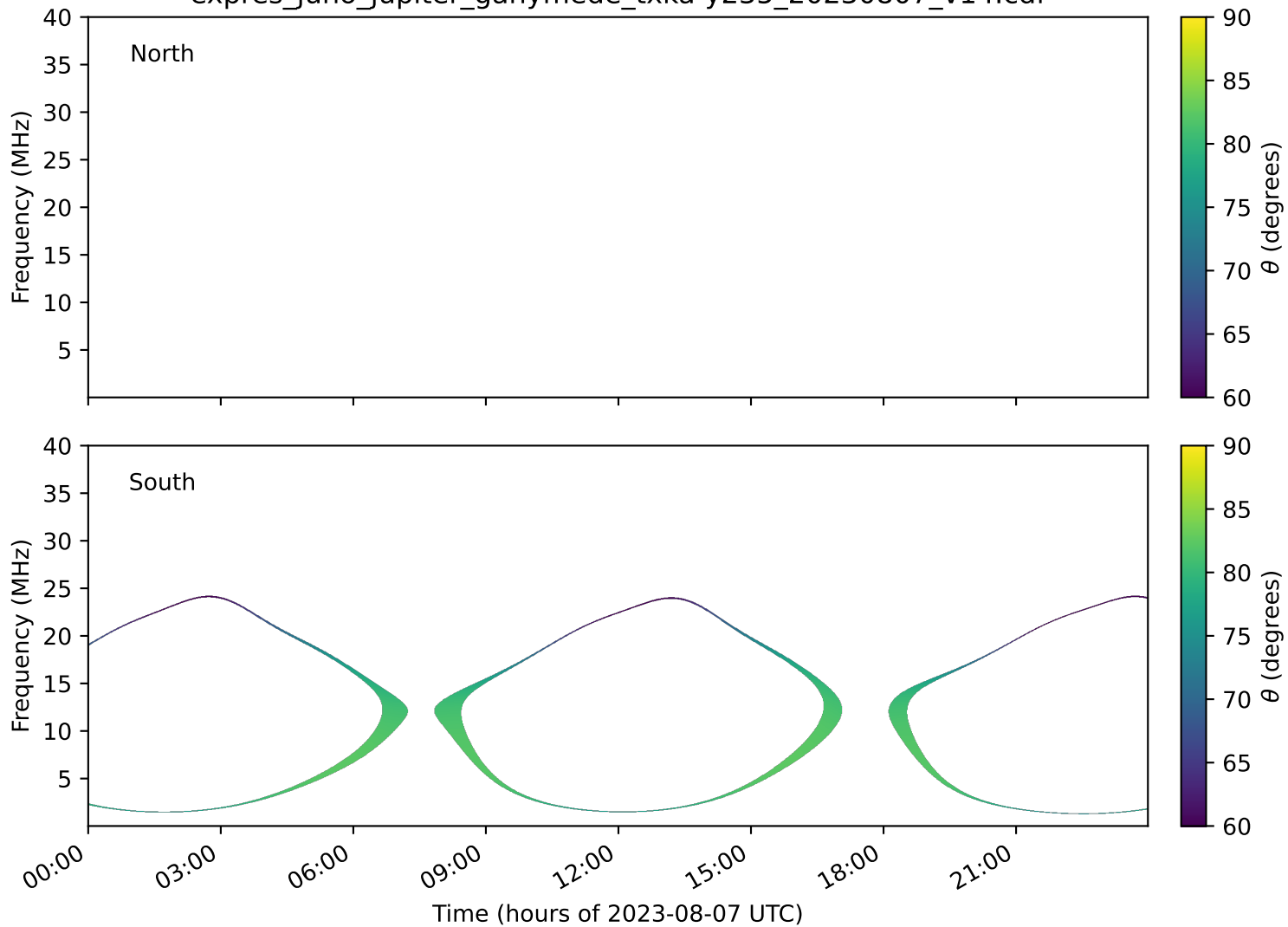
expres_juno_jupiter_ganymede_txka-y235_20230807_v14.cdf
