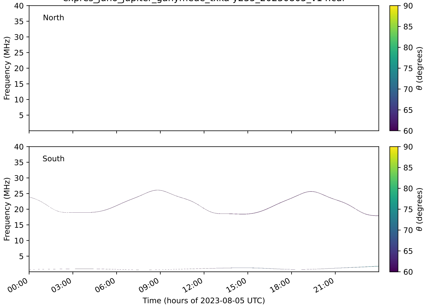
expres_juno_jupiter_ganymede_txka-y235_20230805_v14.cdf
