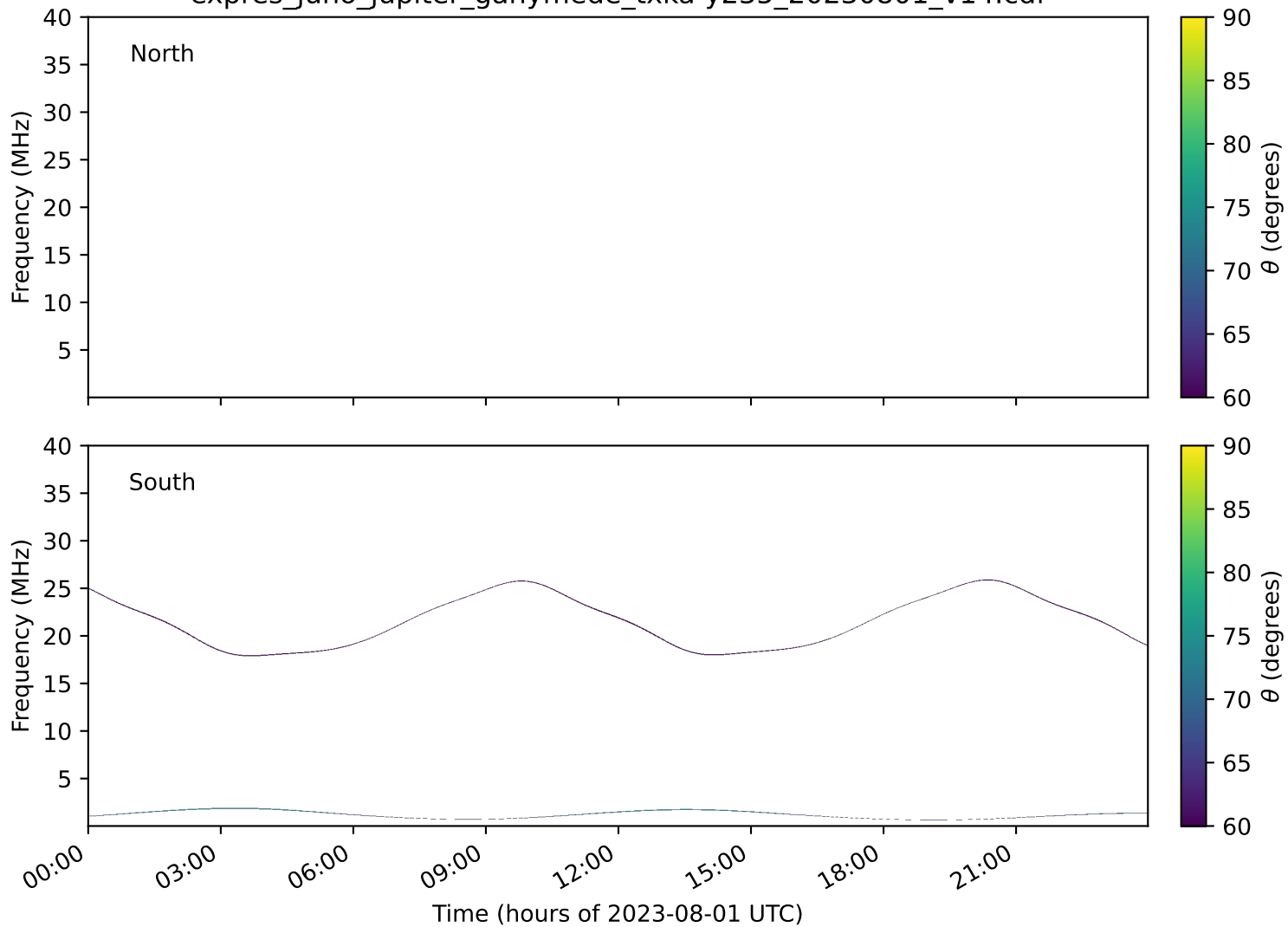
expres_juno_jupiter_ganymede_txka-y235_20230801_v14.cdf
