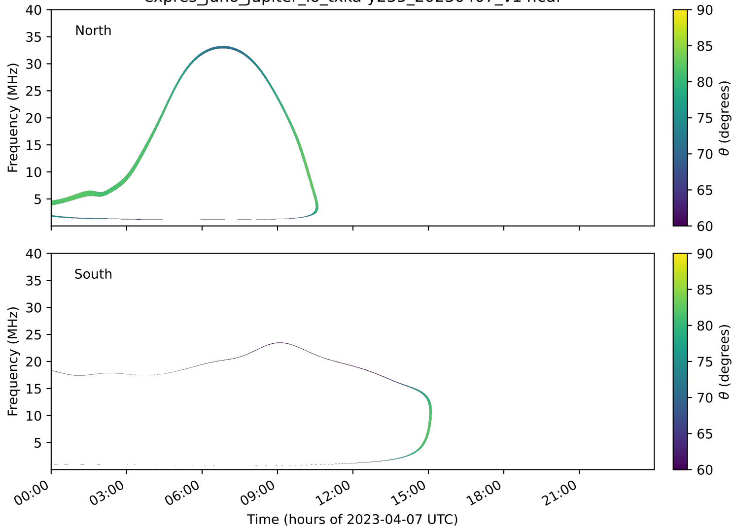
expres_juno_jupiter_io_txka-y235_20230407_v14.cdf
