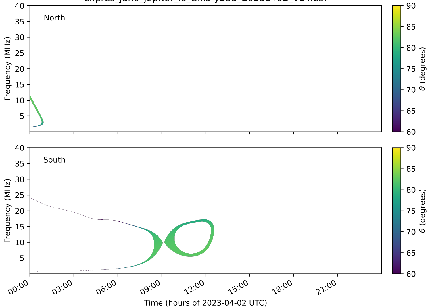
expres_juno_jupiter_io_txka-y235_20230402_v14.cdf
