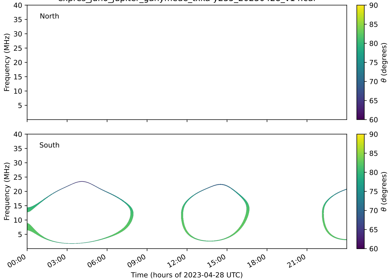
expres_juno_jupiter_ganymede_txka-y235_20230428_v14.cdf
