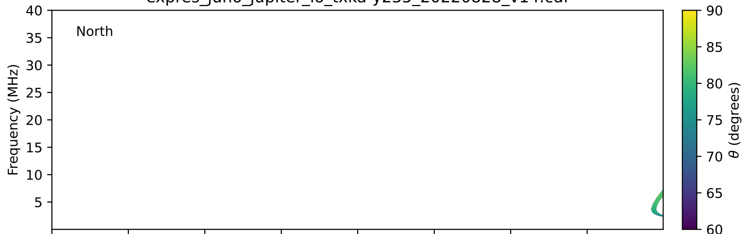
expres_juno_jupiter_io_txka-y235_20220828_v14.cdf
