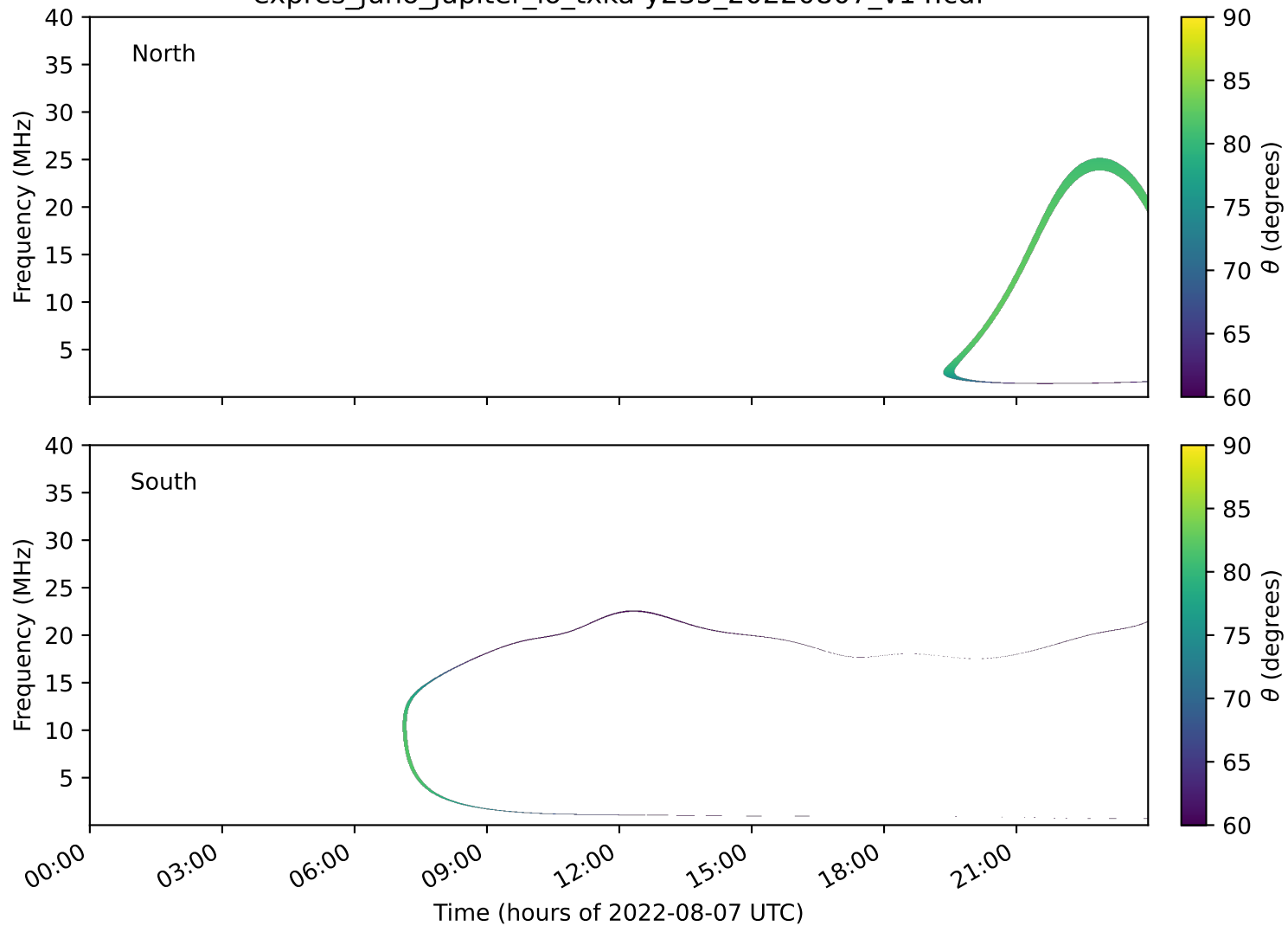
expres_juno_jupiter_io_txka-y235_20220807_v14.cdf
