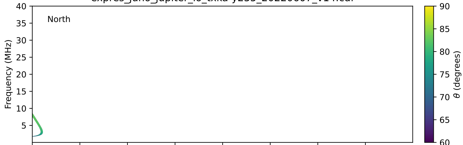
expres_juno_jupiter_io_txka-y235_20220607_v14.cdf
