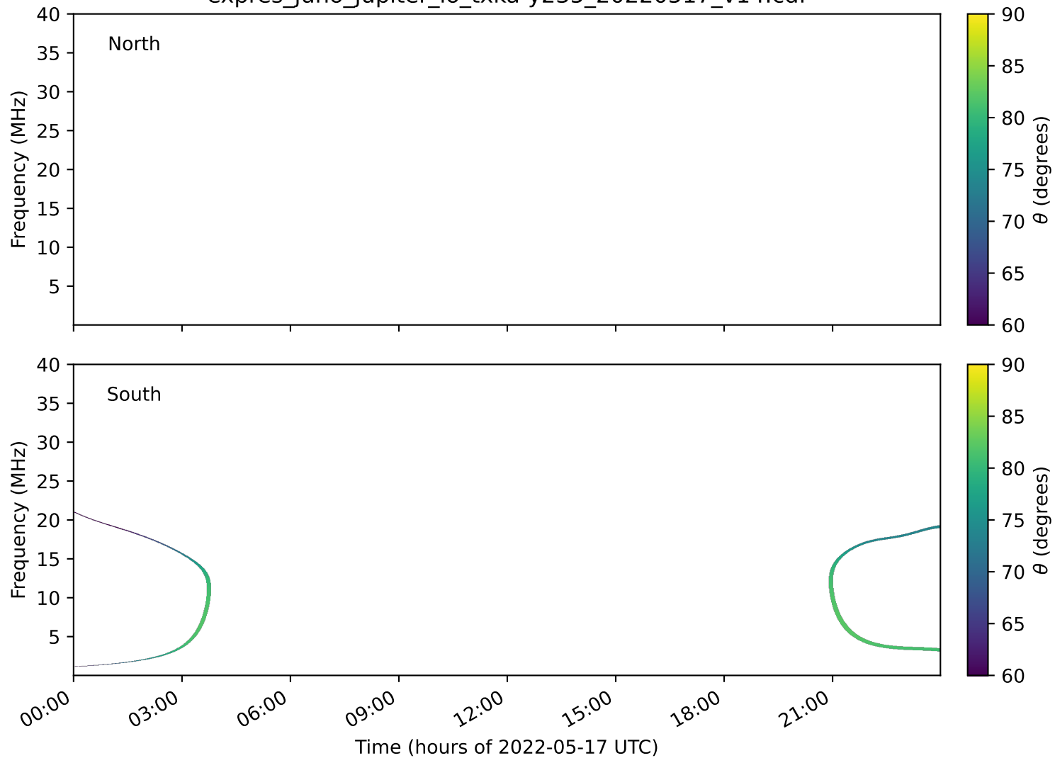
expres_juno_jupiter_io_txka-y235_20220517_v14.cdf
