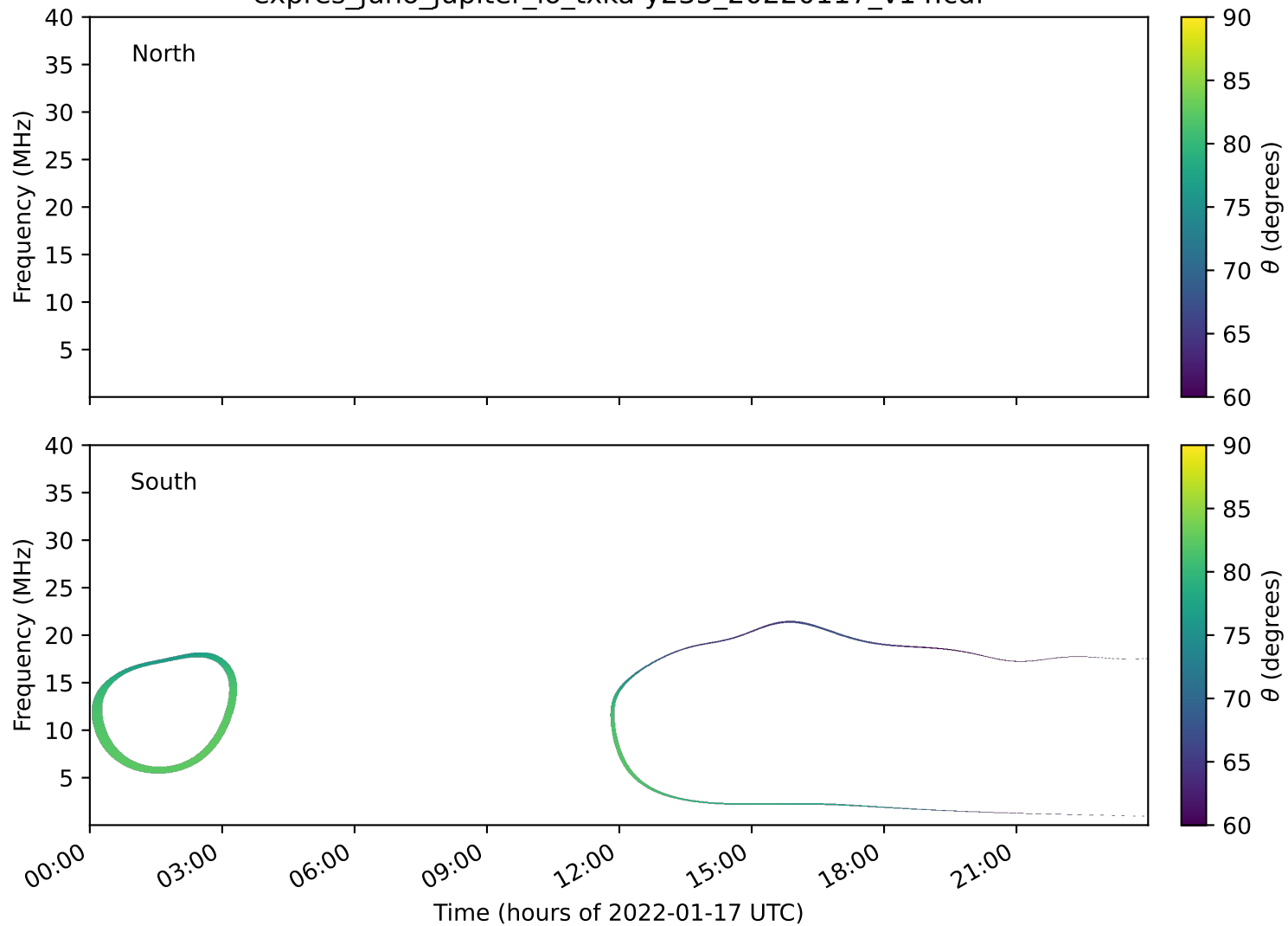
expres_juno_jupiter_io_txka-y235_20220117_v14.cdf
