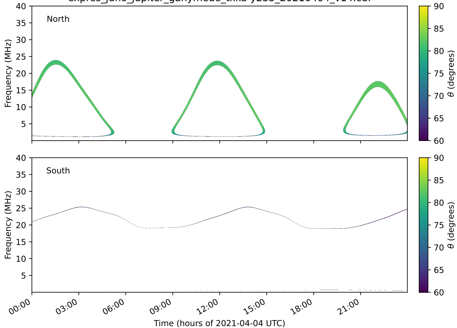
expres_juno_jupiter_ganymede_txka-y235_20210404_v14.cdf
