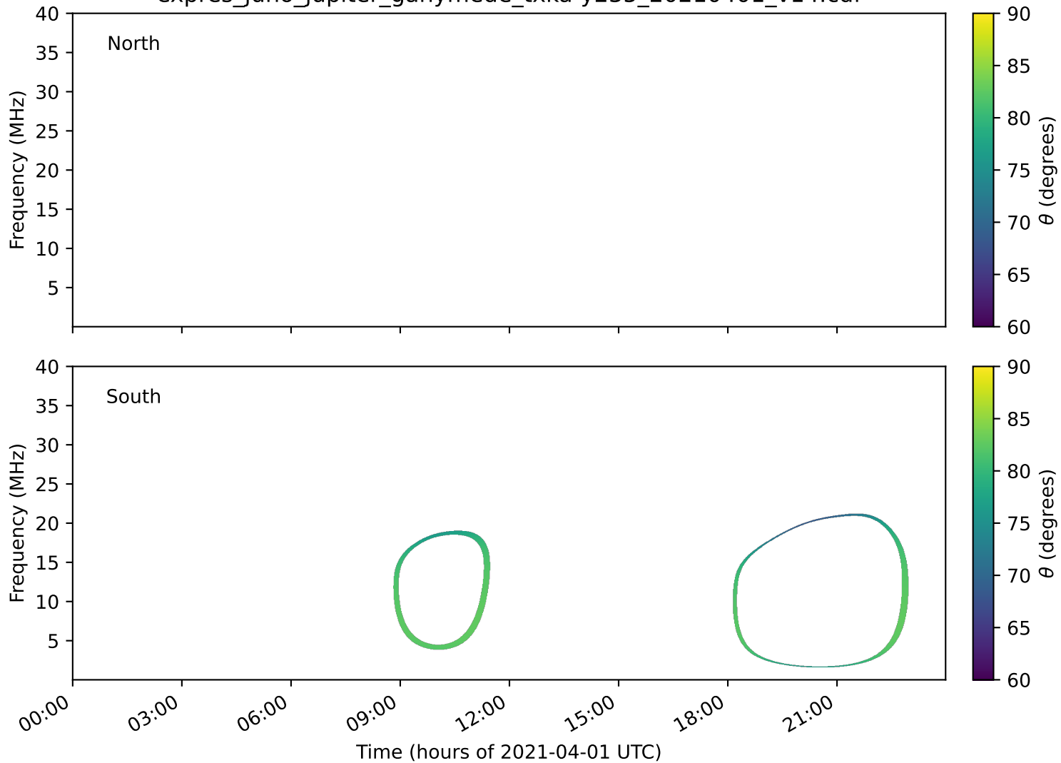
expres_juno_jupiter_ganymede_txka-y235_20210401_v14.cdf
