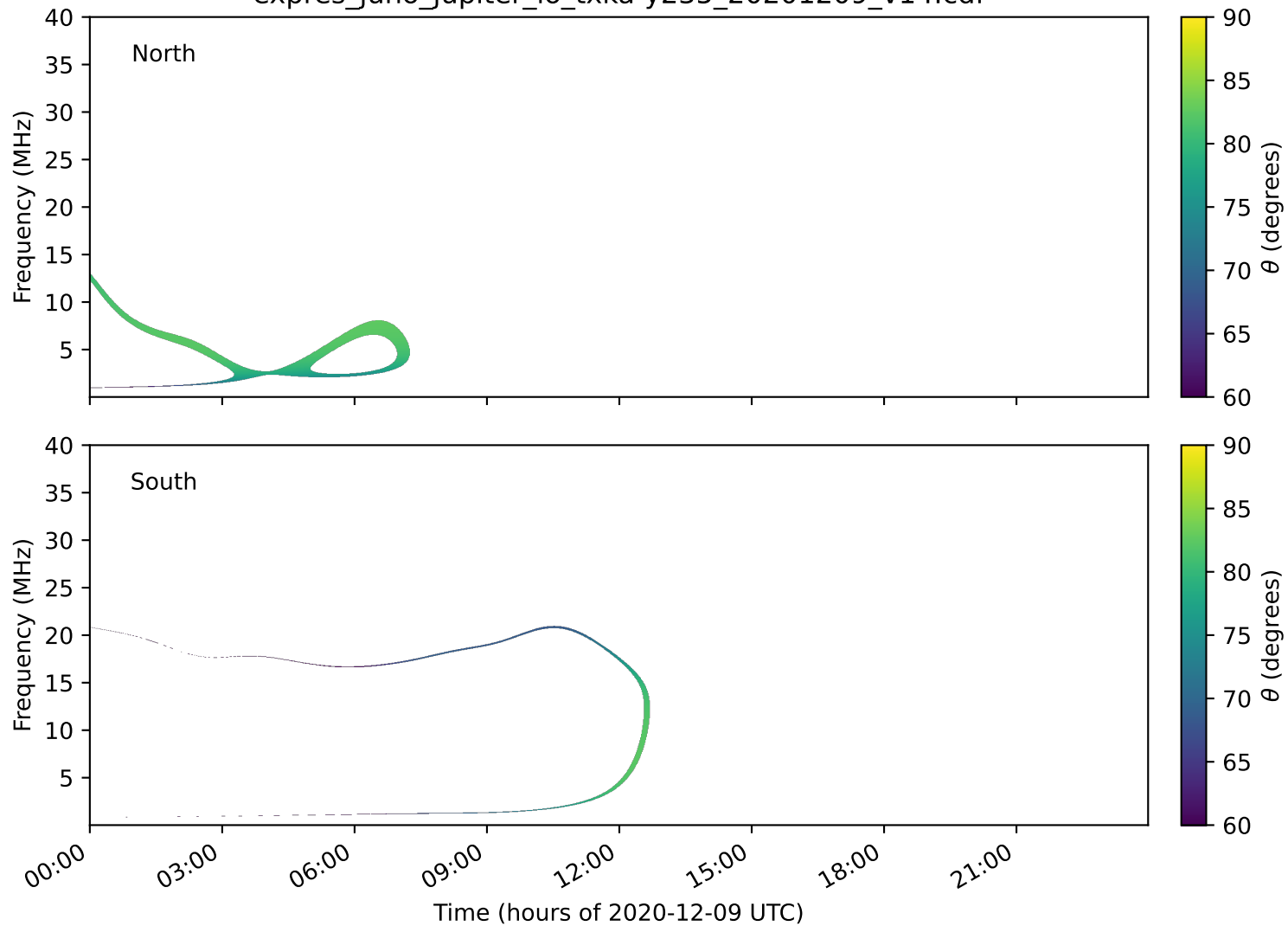
expres_juno_jupiter_io_txka-y235_20201209_v14.cdf
