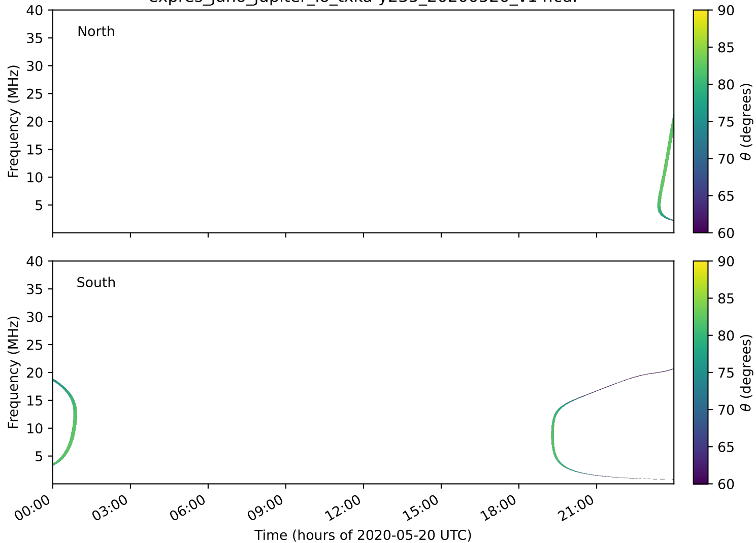
expres_juno_jupiter_io_txka-y235_20200520_v14.cdf
