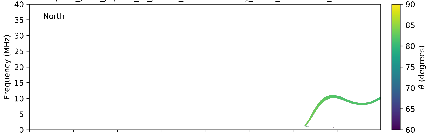
expres_juno_jupiter_io_jrm09_lossc-wid1deg_3kev_20191012_v01.cdf
