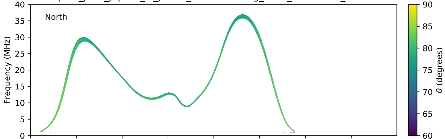
expres_juno_jupiter_io_jrm09_lossc-wid1deg_3kev_20191011_v01.cdf
