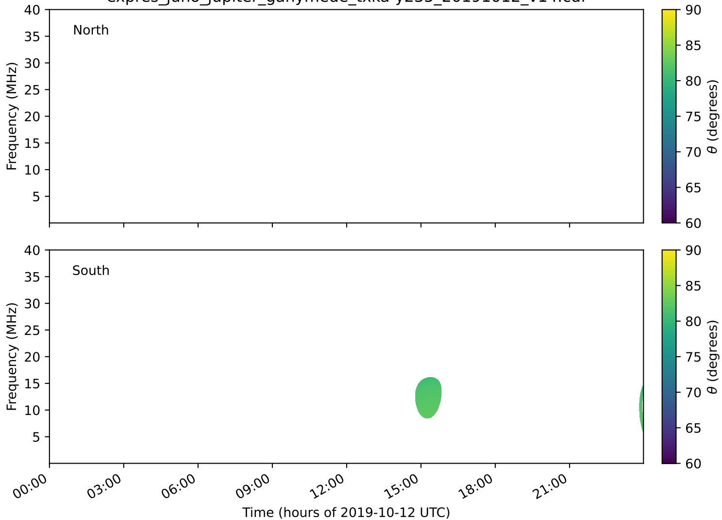
expres_juno_jupiter_ganymede_txka-y235_20191012_v14.cdf
