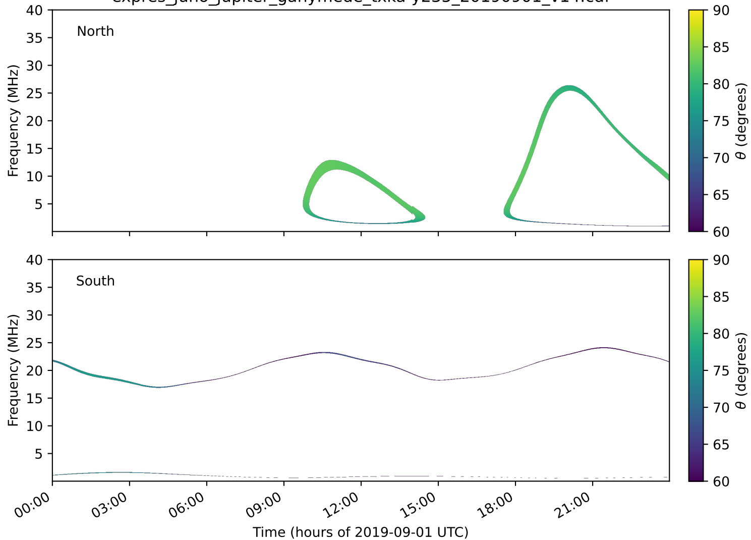
expres_juno_jupiter_ganymede_txka-y235_20190901_v14.cdf
