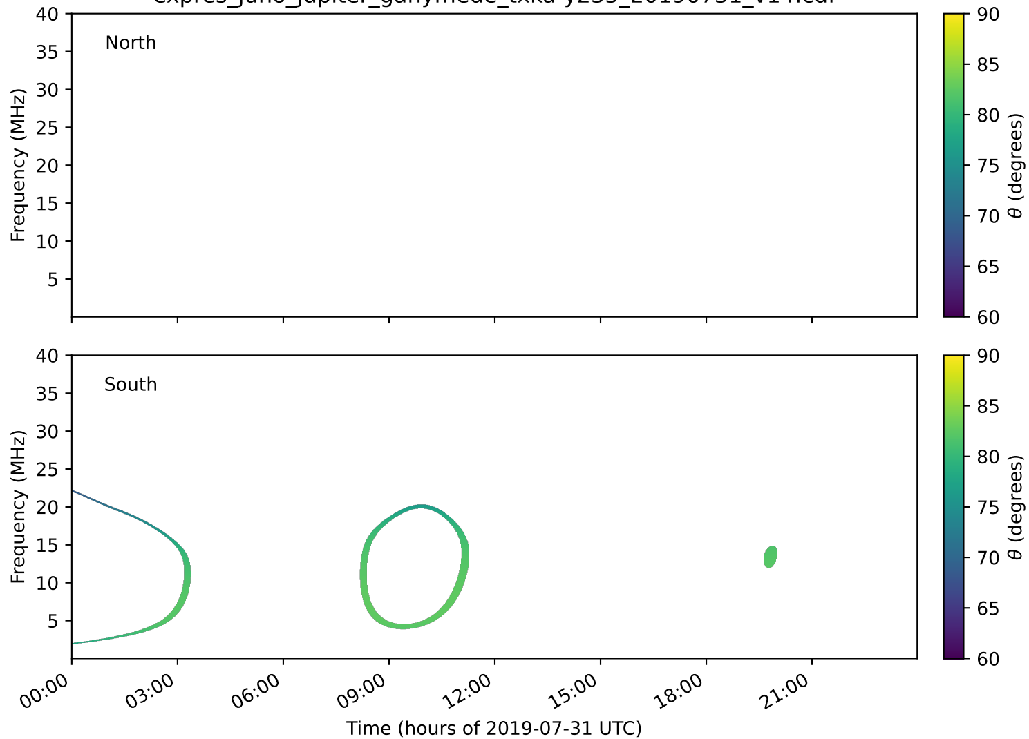
expres_juno_jupiter_ganymede_txka-y235_20190731_v14.cdf
