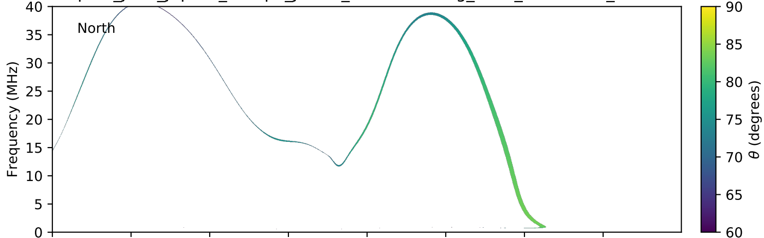
expres_juno_jupiter_europa_jrm09_lossc-wid1deg_3kev_20190209_v01.cdf
