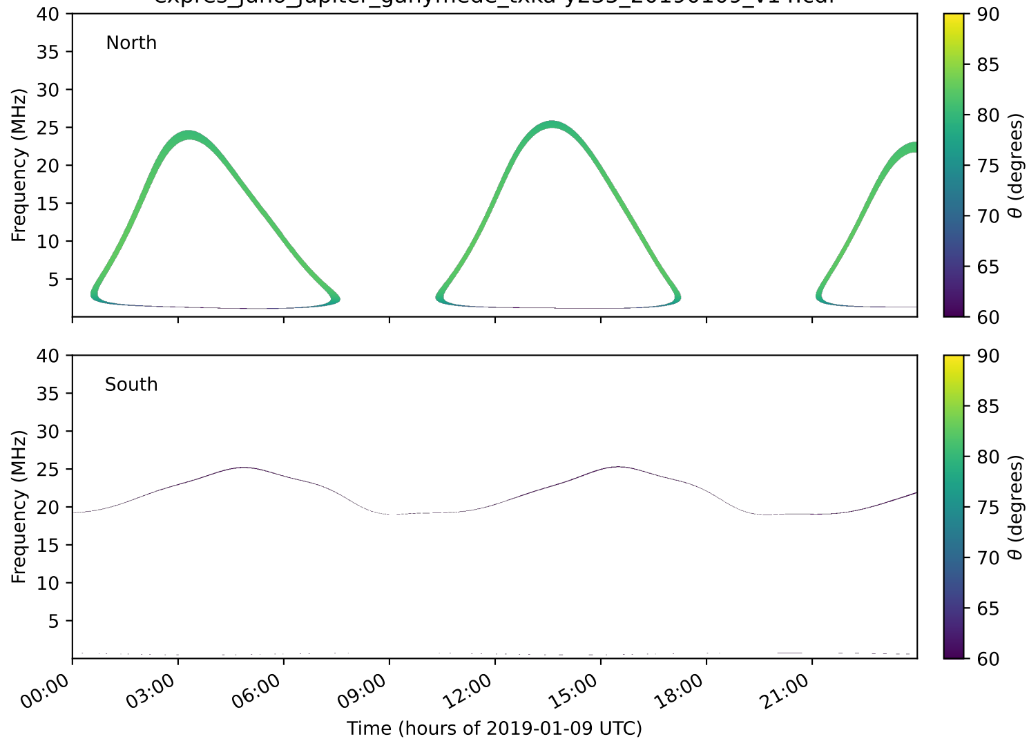
expres_juno_jupiter_ganymede_txka-y235_20190109_v14.cdf
