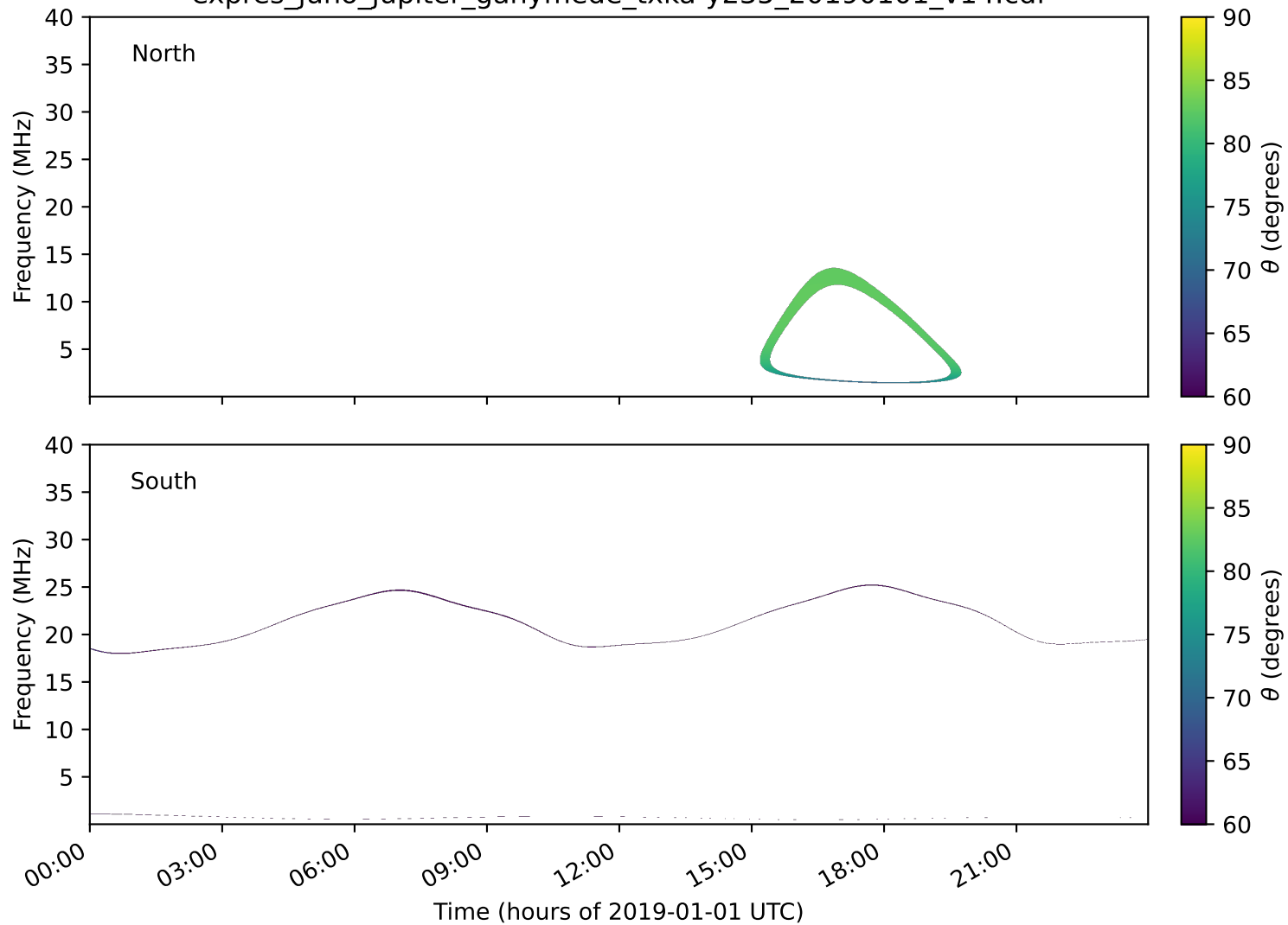
expres_juno_jupiter_ganymede_txka-y235_20190101_v14.cdf
