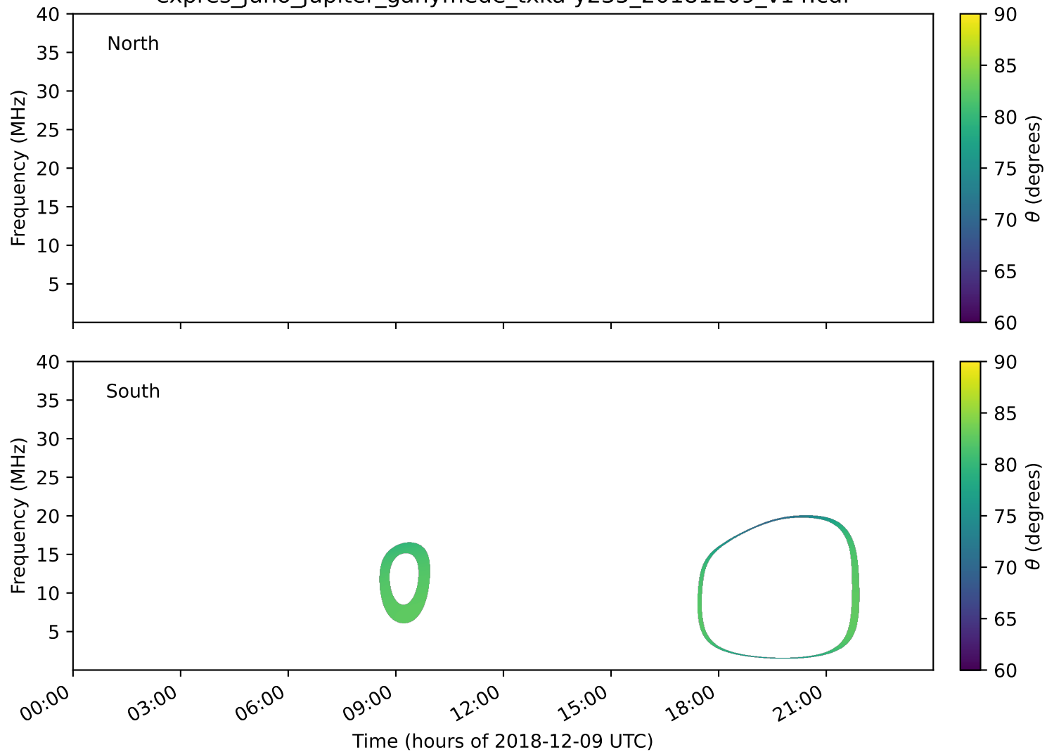
expres_juno_jupiter_ganymede_txka-y235_20181209_v14.cdf
