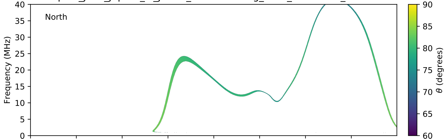
expres_juno_jupiter_io_jrm09_lossc-wid1deg_3kev_20180805_v01.cdf
